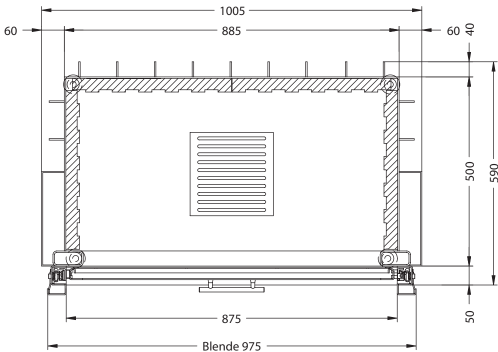
Horizontalschnitt M~1:10
